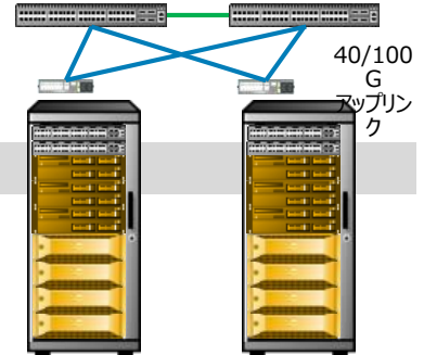
10GbE サーバ/ストレージ 10GBaseT サーバ/ストレージ
